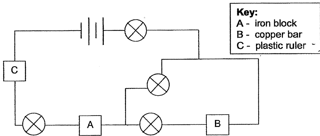
circuit Y
